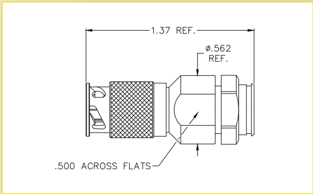
ZMA MALE (ZXPS-2801)
