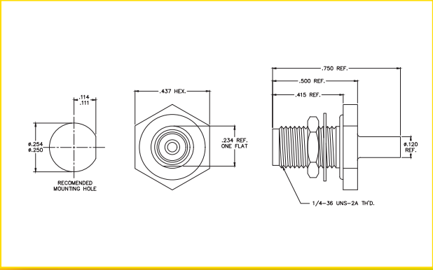
SMA FEMALE BULKHEAD (SJBD-TPRF085)
