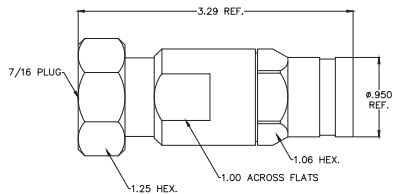
7/16 DIN MALE (716PS-7506)
