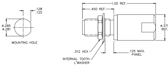
SMA FEMALE BULKHEAD (SJB-TPRF141)
