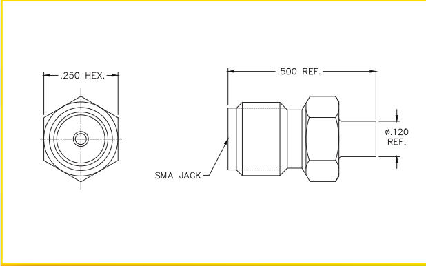
SMA FEMALE (SJSD-TPRF085)
